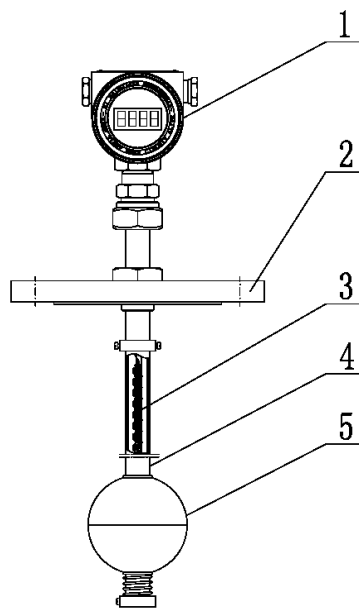
图 1 产品主要结构
