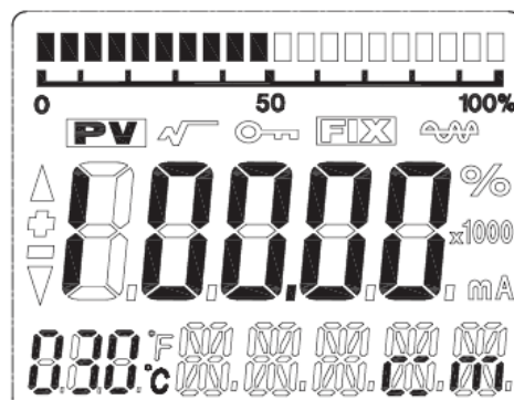
图 7-2 主变量显示
