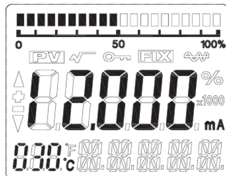
图 7-2 电流显示
