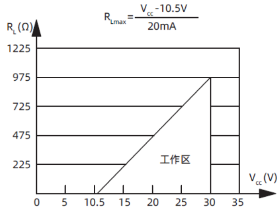
图 2 负载特性图
